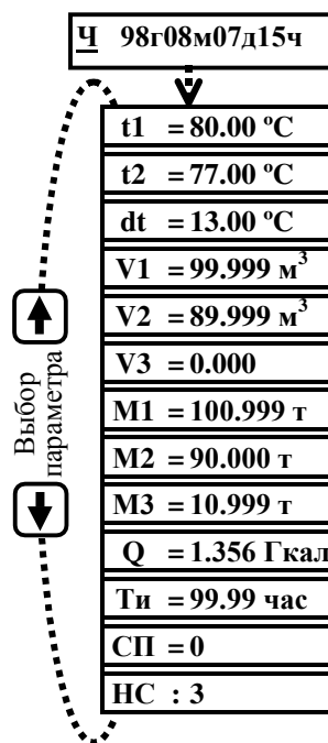
Рисунок 3.6 – Структура раздела АРХ
