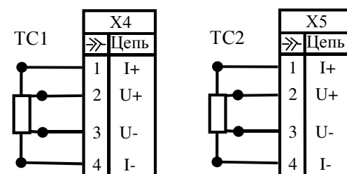
Рисунок 5.8 – Подключение ТС
