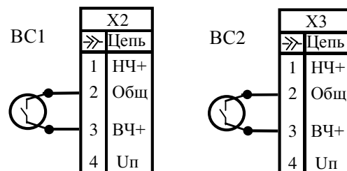
Рисунок 5.6 – Подключение без питания ВС к моделям 05-08
