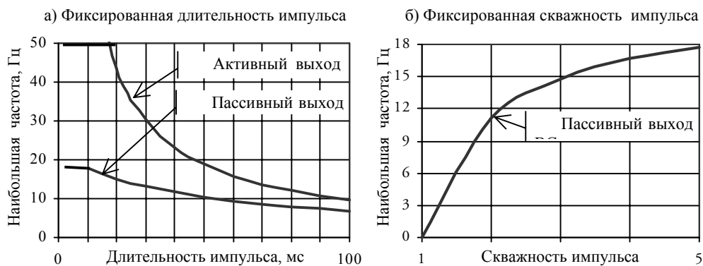
Рисунок 6.1 – Набольшая частота у моделей 01-04 и входа НЧ моделей 05-08
